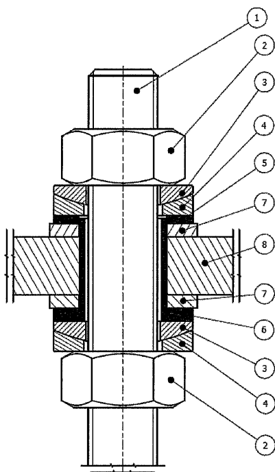
Schemat 1 Mocowanie osprzętu dla fundamentów palowych przeznaczonych pod słupy bramek trakcyjnych i słupów przestrzennych przez dwa tory
