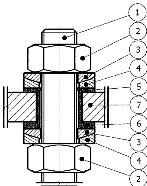
Schemat 2 Mocowanie osprzętu dla fundamentów palowych przeznaczonych pod konstrukcje wsporcze sied trakcyjnej
