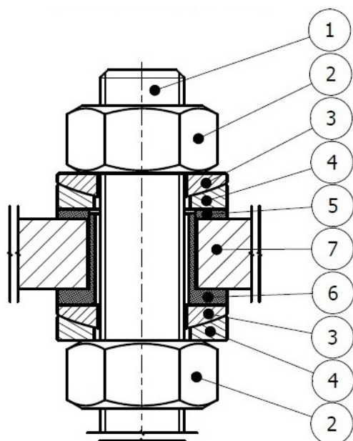
Schemat 2 Mocowanie osprzętu dla fundamentów paliowych przeznaczonych pod konstrukcję wsporcze sieci trakcyjnej
