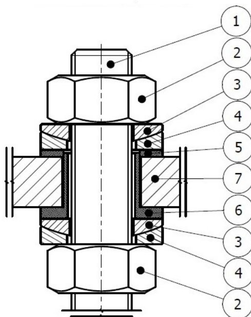
Schemat 2 Mocowanie osprzętu dla fundamentów palowych przeznaczonych pod konstrukcje wsporcze sieci trakcyjnej
